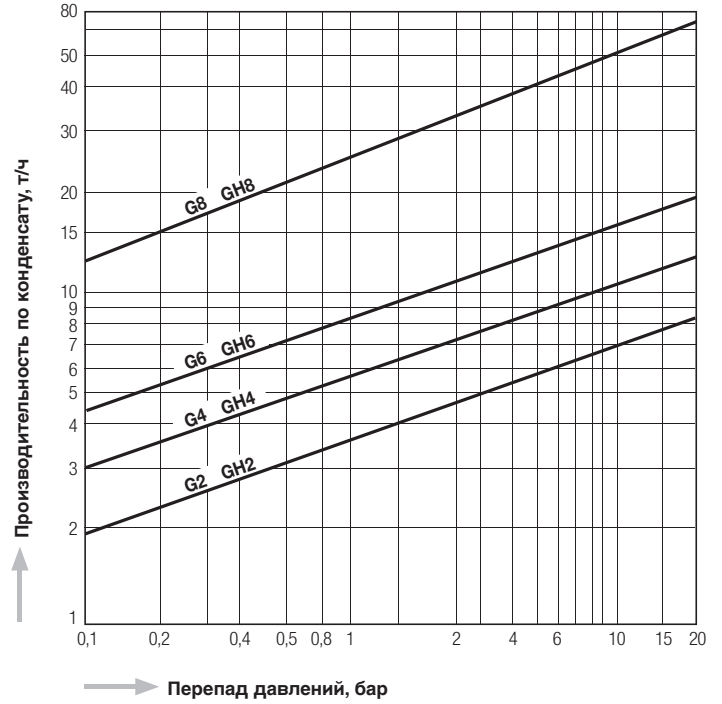
График производительности
